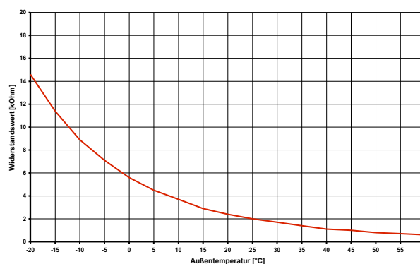
Fig. 8.2: Courbe caractéristique de la sonde NTC-2 selon DIN 44574 Sonde de température extérieure
