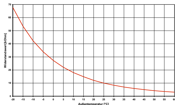
Abb. 9.1: Fühlerkennlinie NTC-10
