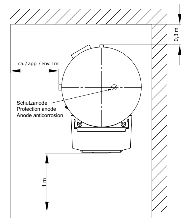
Abb. 5.1: Abstände Inneneinheit
