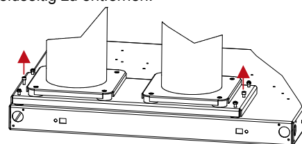
Transportsicherung entfernen/einschrauben
