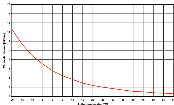
Afb. 7.2: Voelerkarakteristiek Norm-NTC-2 volgens DIN 44574 buitentemperatuurvoeler
