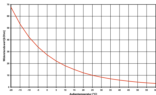
Afb. 7.1: Voelerkarakteristiek NTC 10
