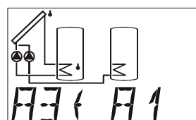
A3 schakelt met A1
