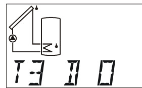
Digitale toestand (digitale ingang)
