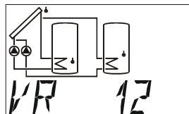
Voorrang A1 voor A2
