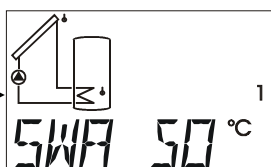
Gewenste waarde abs.waardereg.
